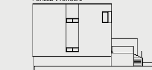
POHLED SEVERNÍ
